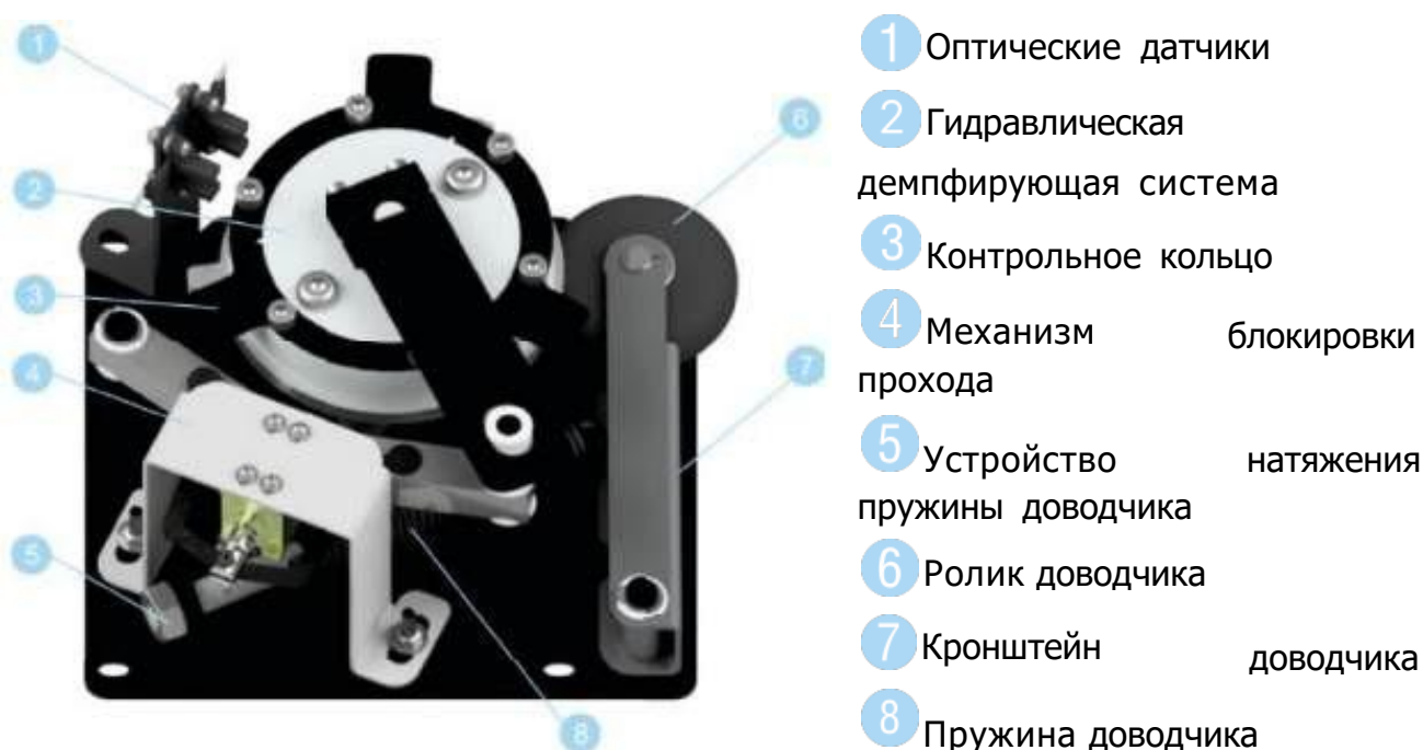
Рисунок 6.2.1. - Устройство механизма турникета
