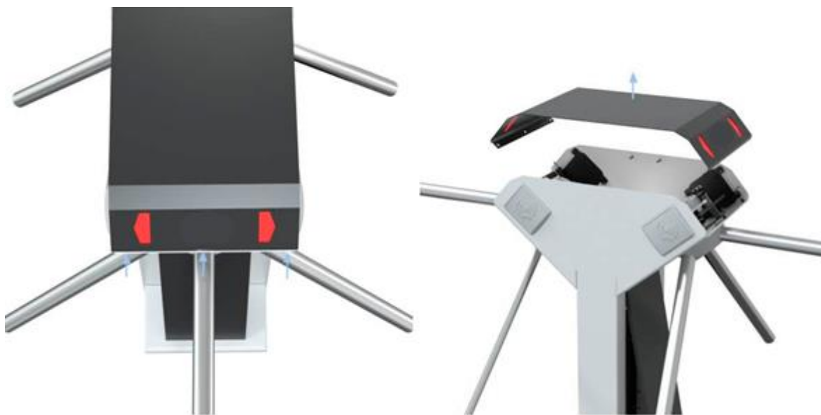
Рисунок 12.1.1 - Демонтаж верхней крышки турникета
