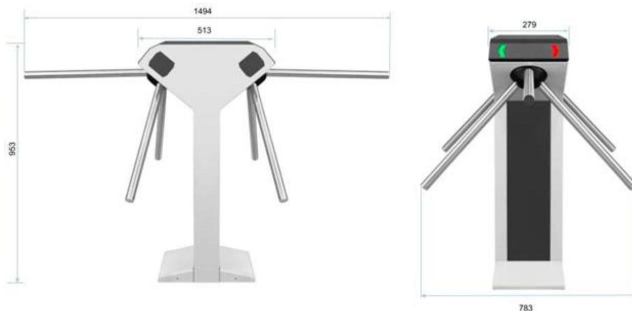
Рисунок 5.1 - Габаритные размеры турникета с планками «TDX-01»
