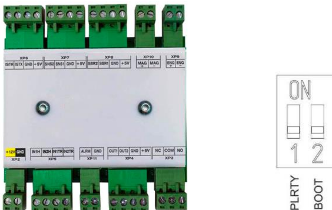
Рисунок 6.3.1 Контроллер управления турникетом «AT-002B» Dip-переключатели
