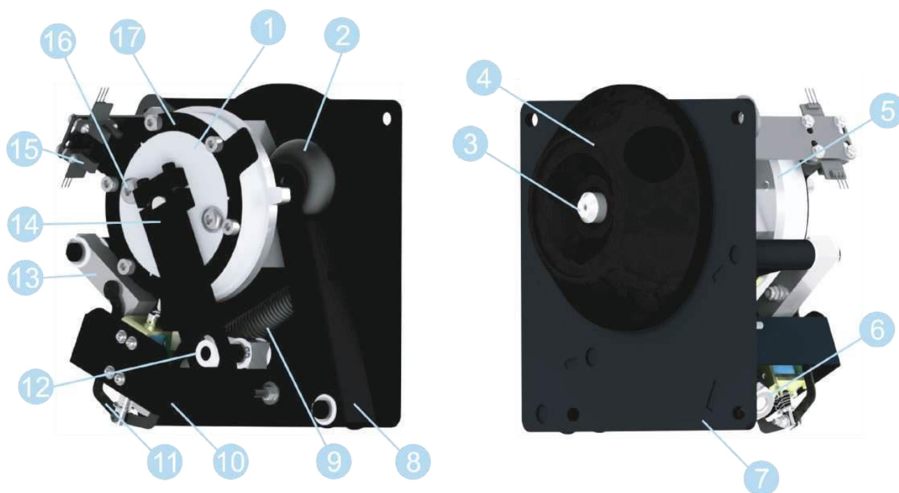
Рисунок 12.2.1 - Расположение узлов механизма турникета AT-010
